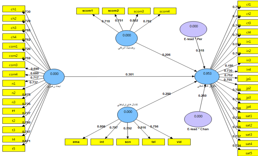
شکل ۱. ضرایب مسیر
