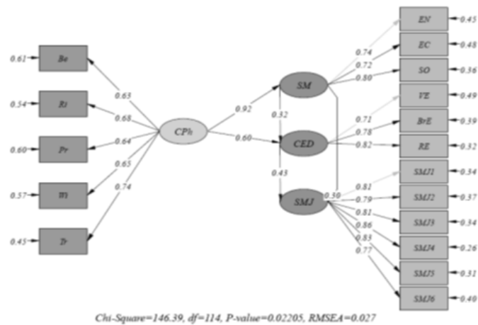
نمودار ۲. مدل ساختاری پژوهش
